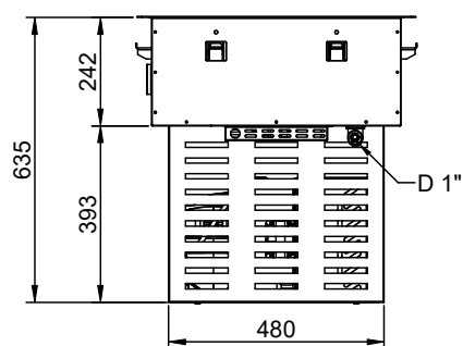
Zij aanzicht
