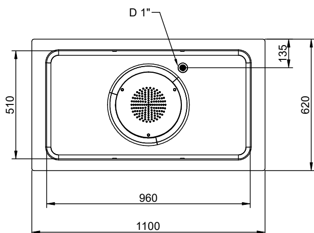
Boven aanzicht
